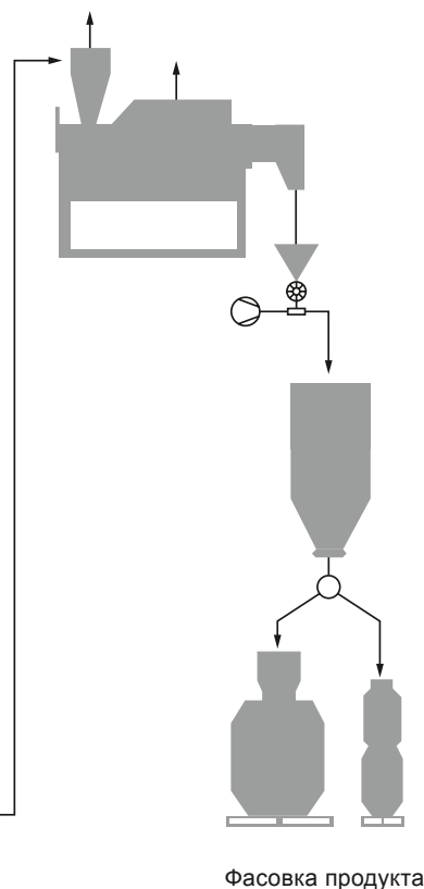
Охладитель гранул
