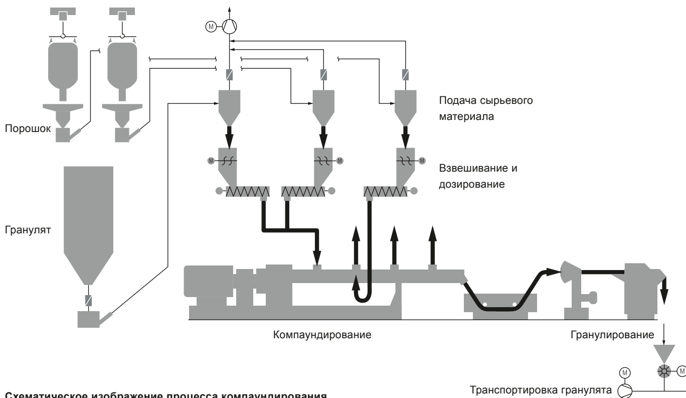
Схематическое изображение процесса компаундирования
